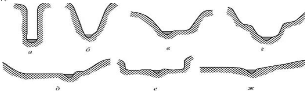
Расми 4. Буриши кундалангии ҷои сохтмони дарғот. а,б,в,г- дарғотҳои кӯҳӣ; д,е,ж- дарғотҳои водигӣ.
