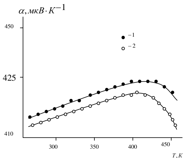
Рис. 3. Температурная зависимость коэффициента термо-э.д.с. соединения In_2Te .
