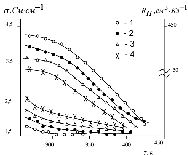
Рис.1. Температурные зависимости электропроводности – (нижние кривые) и коэффициента Холла (верхние кривые) соединения \text{In}_2\text{Te} .
