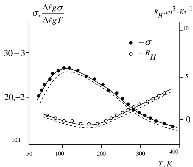
Рис.2. Температурная зависимость электропроводности и коэффициента Холла In_2Te .
